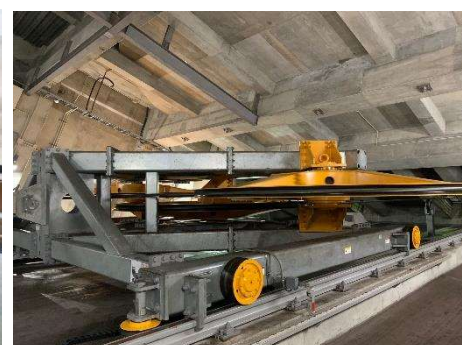
箱根ロープウェイの運転指令所・技術区 ロープを動かすモーター
